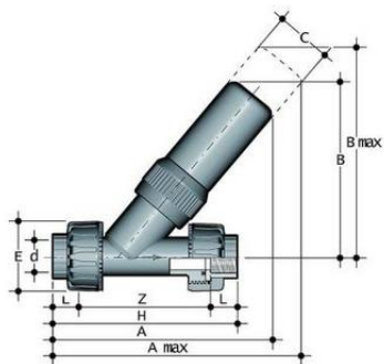
Угловой предохранительный клапан SV PBX с резьбовыми окончаниями, FKM, FIP R1/2" (DN15)
