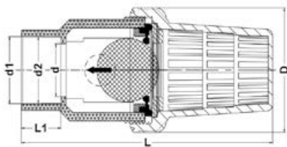
Донный клапан IVZ ПВХ с муфтовыми окончаниями, FKM, FIP d75 (DN65)
