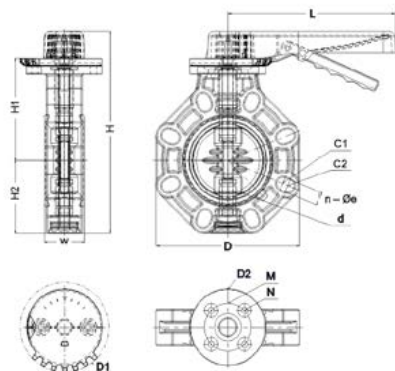
Затвор дисковый ПВХ с рукояткой промышленного применения FKM IPS d225
