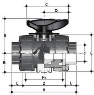
Шаровой кран ПВХ для регулирования потока VKR с муфтовыми окончаниями, FKM, FIP d20 (DN15)
