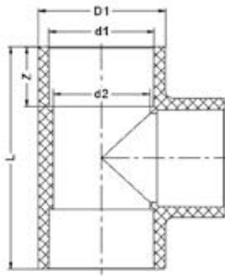
Тройник для раструбной сварки 90° PP-H IPS d110 PN10
