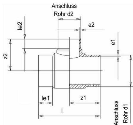
Тройник редукционный PP-H Simona (PN6) 180x110 SDR17.6 PN6
