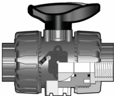
Шаровой кран ПВХ промышленного применения VKD с резьбовыми окончаниями, EPDM, FIP R2" (DN50)
