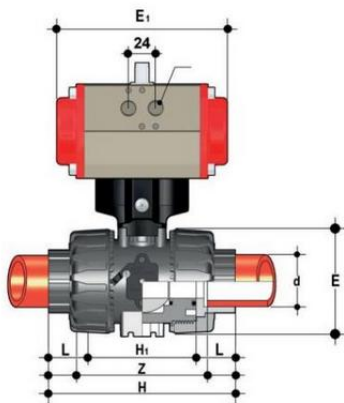
Шаровой кран VKD ПВДФ с пневмоприводом ДВД с муфтовыми окончаниями d32 (DN25)
