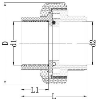
Муфта разборная с ВР, РР-Н IPS d50 PN10
