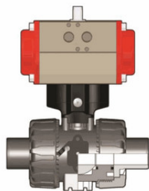
Шаровой кран VKD ПВДФ с пневмоприводом НО с втулочными окончаниями d40 (DN32)
