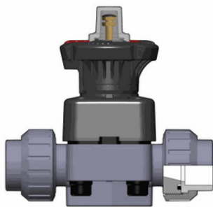
Мембранный клапан DKLUIV PBX с разборными муфтовыми окончаниями, EPDM, FIP d32 (DN25)
