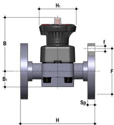
Мембранный клапан DKOV PBX с фланцевыми окончаниями, EPDM, FIP d75 (DN65)
