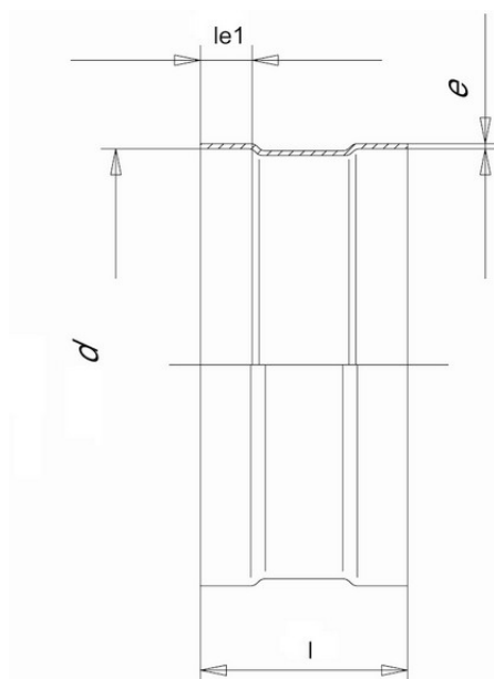
Муфта PPs d180
