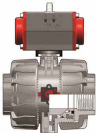
Шаровой кран VKD ПВХ с пневмоприводом НЗ с резьбовыми окончаниями, FKM, FIP R4" (DN90)
