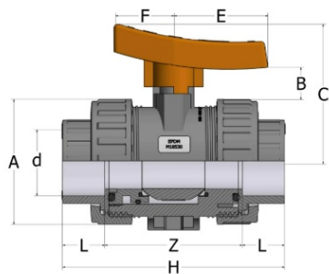
Шаровой кран ПВХ промышленного применения с муфтовыми окончаниями, EPDM, Comer d40 (DN32)
