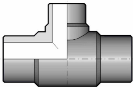
Тройник редукционный для стыковой сварки PP-H FIP 160x75 SDR11 PN6
