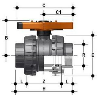
Шаровой кран общего применения VXE ХПВХ с резьбовыми окончаниями, DN65-100 R3" (DN80)
