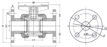
Кран шаровой промышленного применения, фланцевые окончания, FKM, IPS d90
