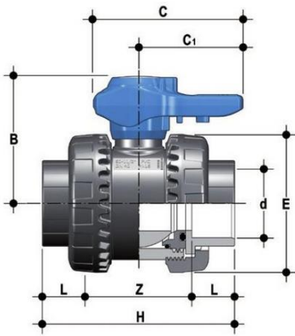
Шаровой кран ПВХ общего применения VEE; муфтовые окончания, EPDM, FIP d32 (DN25)
