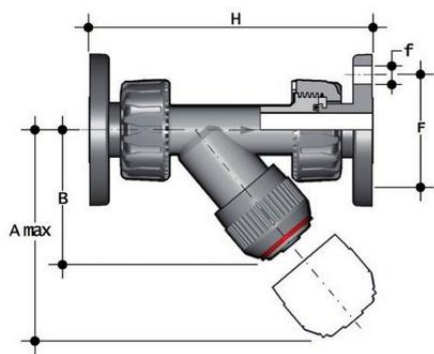
Грязевой фильтр RVUOM с фланцевыми окончаниями (уплотнение FKM) PP-H d63 (DN50)
