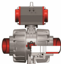
Шаровой кран VKD ПВДФ с пневмоприводом ДвД с муфтовыми окончаниями d110 (DN90)
