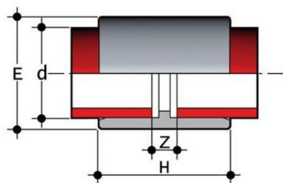
Муфта соединительная ПВДФ d25 SDR21 PN16
