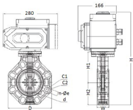
Дисковый затвор IFK ПВДФ с электрическим приводом 24V DC, EPDM, IPS d160 (DN150)
