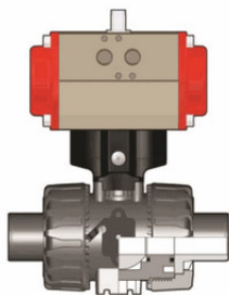
Шаровой кран VKD с пневмоприводом НО с втулочными окончаниями (уплотнение EPDM) PP-H d40 (DN32)
