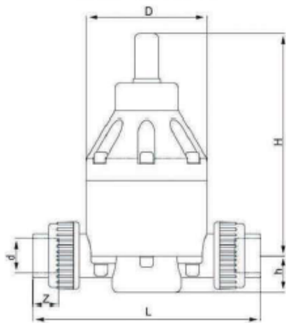
Клапан поддержания давления ПВХ с муфтовыми окончаниями, IPS d20 (DN15)
