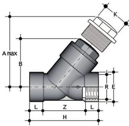
Угловой обратный клапан VRFV ПВХ с резьбовыми окончаниями, EPDM, FIP R3" (DN80)
