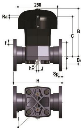
Мембранный клапан VM ПВДФ с пневмоприводом НО с втулочными окончаниями d90 (DN80)
