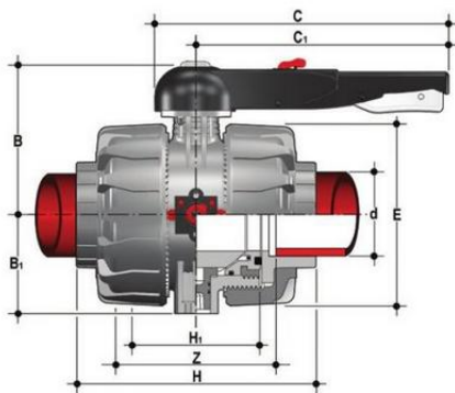
Шаровой кран VKD ПВДФ с муфтовыми окончаниями, DN65-110 d110 (DN100)
