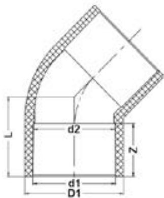
Отвод для раструбной сварки 45° PP-H IPS d32 PN10
