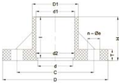
Жесткий фланец ХПВХ IPS (Model A) d90 PN16
