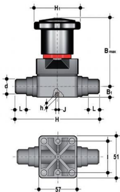
Компактный мембранный клапан CMDC ХПВХ с втулочными окончаниями d20 (DN15)
