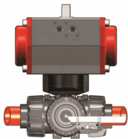
3-х ходовой шаровой кран ТКД с пневмоприводом ДвД с муфтовыми окончаниями, Т-шар (уплотнение FKM) PP-H d16 (DN10)
