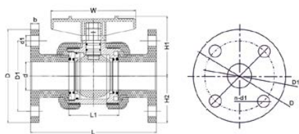
Шаровой кран IVKD ПВДФ с фланцевыми окончаниями (FKM) d20 (DN15)
