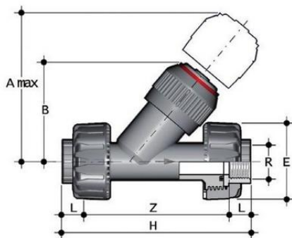
Угловой обратный клапан VRUFV ПВХ с резьбовыми окончаниями, EPDM, FIP R3/4" (DN20)
