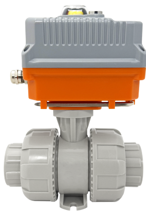
Шаровой кран IVKD ПП-гомополимер с эл.приводом 24V DC, муфтовые окончания, EPDM, IPS d20 (DN15)
