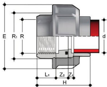
Разборная муфта с ВР, раструбная сварка РР-Н (EPDM) FIP 50x1 1/2 PN10
