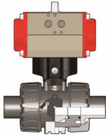
Шаровой кран VKD ПВХс пневмоприводом НЗ с втулочными окончаниями, FKM, FIP d40 (DN32)
