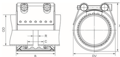
Муфта соединительная Straub-METAL-GRIP Ø30.0-219.1, NBR, W5 d159
