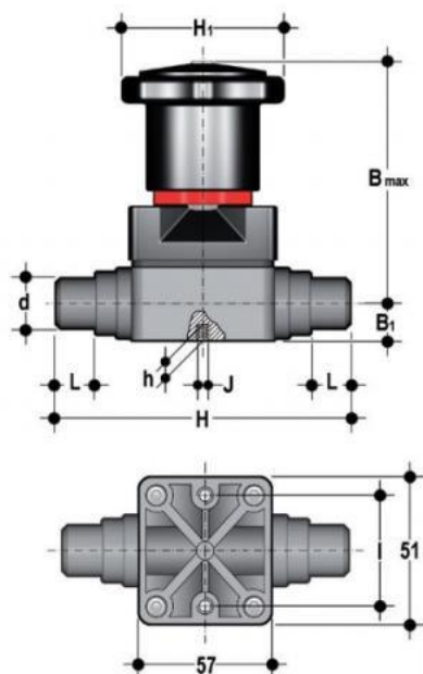
Компактный мембранный клапан CMDV PBX с втулочными окончаниями, FKM, FIP d20 (DN15)
