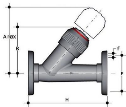
Угловой обратный клапан VROV PBX с фланцевыми окончаниями, EPDM, FIP d20 (DN15)
