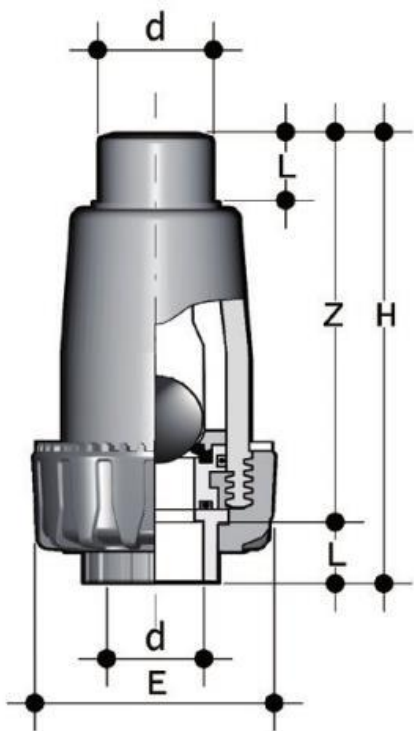
Шаровой обратный клапан SR ПВДФ, муфтовые окончания d63 (DN50)
