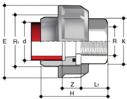
Муфта разборная переходная PP-H / нерж.сталь, ВР, (FKM) FIP 32x1 PN10
