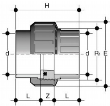
Муфта разборная клеевая ПВХ FIP d20
