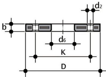
Свободный фланец РР-Н FIP (PN16) d315 PN16
