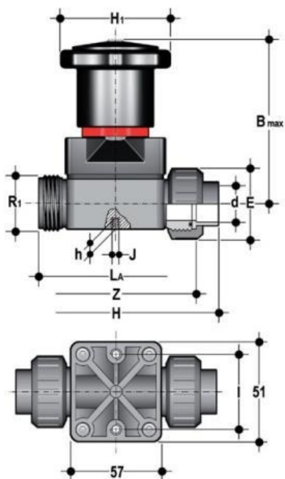
Компактный мембранный клапан CM с разборными муфтовыми окончаниями (уплотнение FKM / мембрана PTFE) PP-H d20 (DN15)
