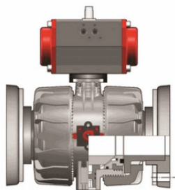
Шаровой кран промышленного применения VKD PBX с пневмоприводом, FIP d75 (DN65)
