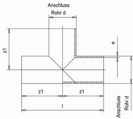
Тройник ПВДΦ 90° (Simona) d160 SDR21 PN16
