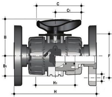
Шаровой кран для регулирования потока VKR с фланцевыми окончаниями (уплотнение FKM) PP-H d63 (DN50)
