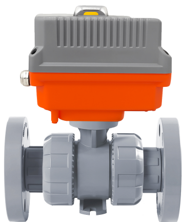
Шаровой кран IVKD ХПВХ с эл.приводом 24V DC, фланцевые окончания d40 (DN32)
