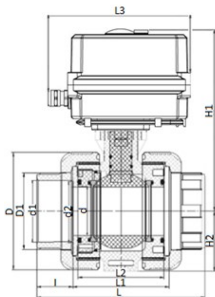
Шаровой кран IVKD ХПВХ с эл.приводом 24V DC, муфтовые окончания d75 (DN65)
